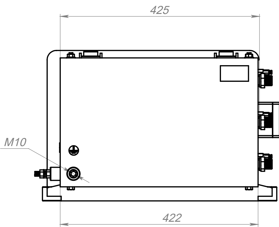
Вид справа
