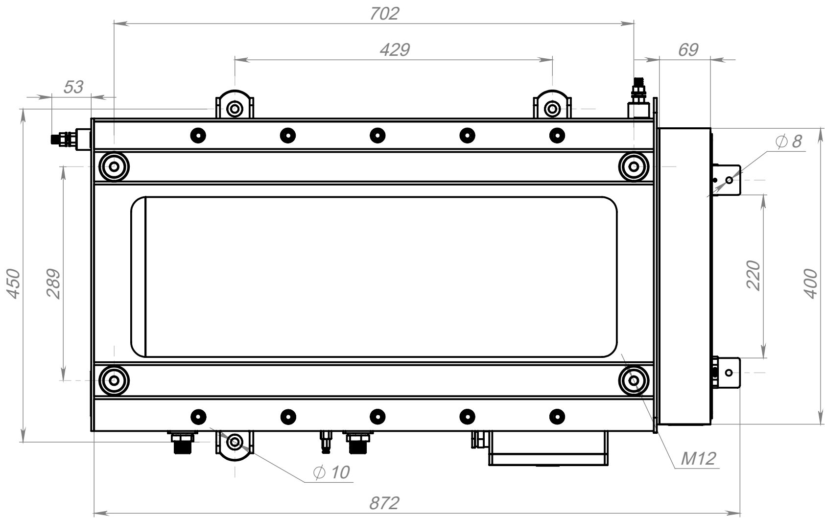
вид сверху
