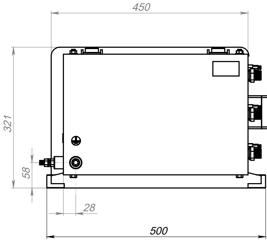
Вид слева
