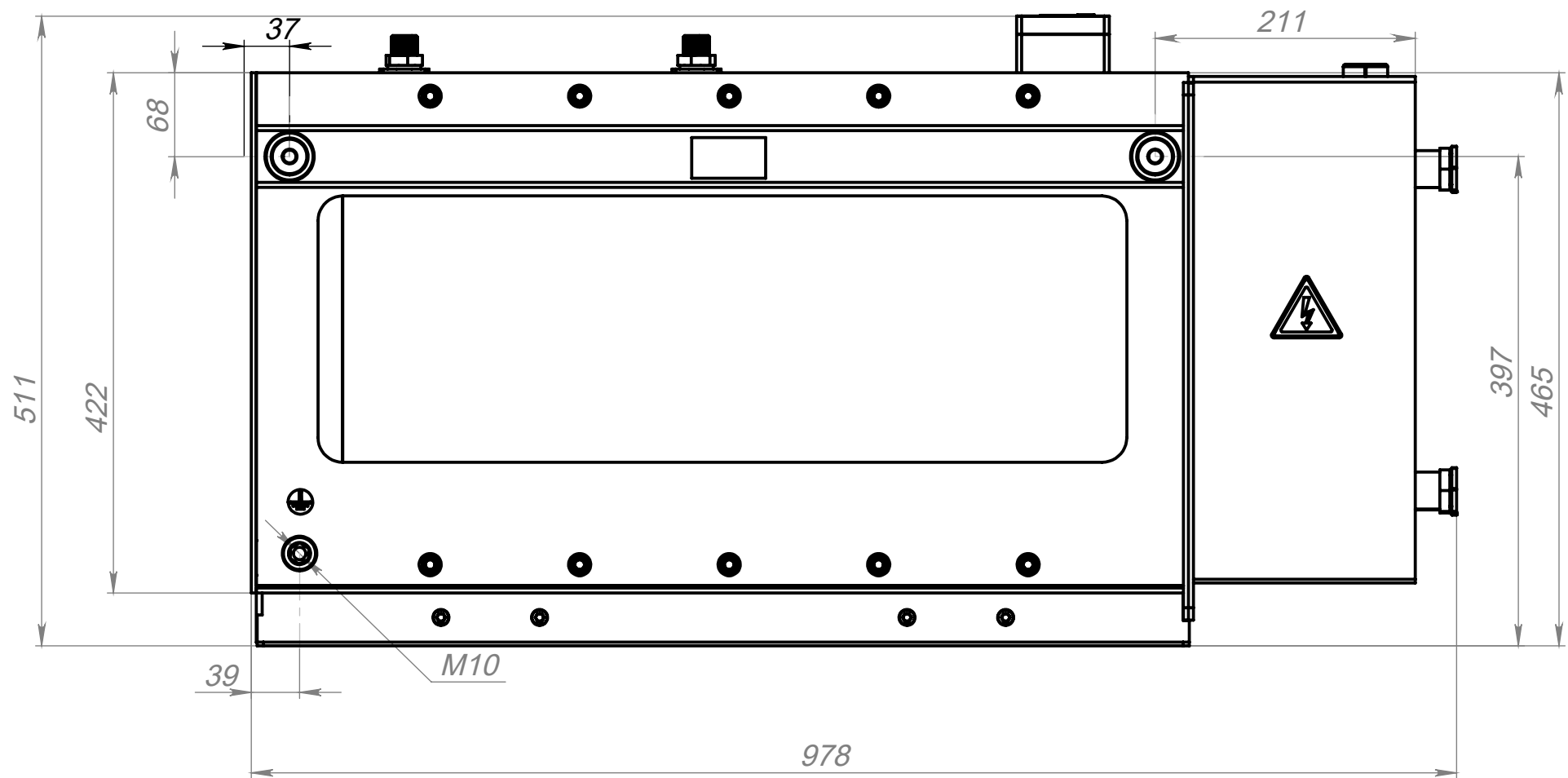
Вид слева
