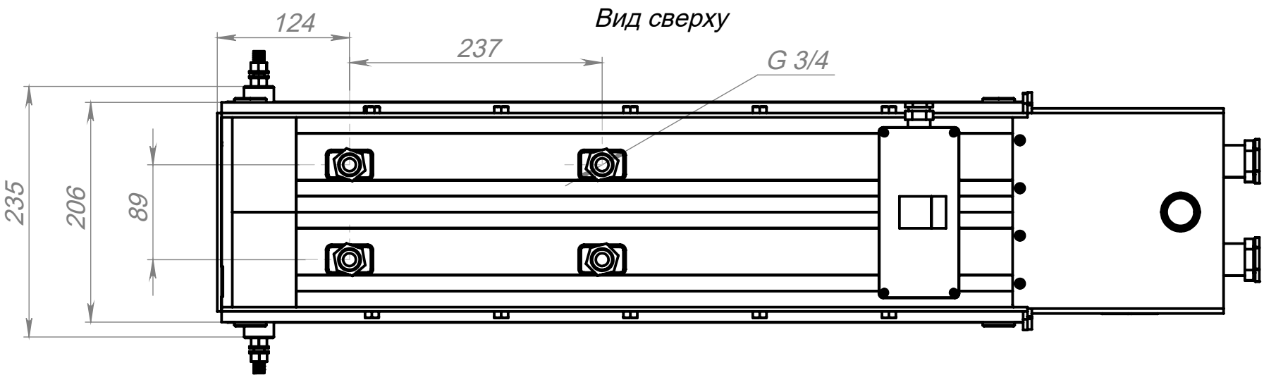
Вид сверху
