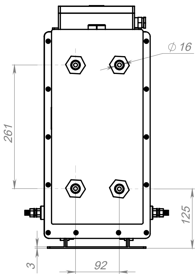
Вид спереди
