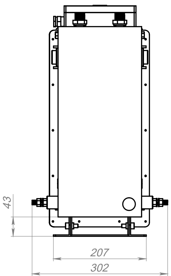
Вид сзади
