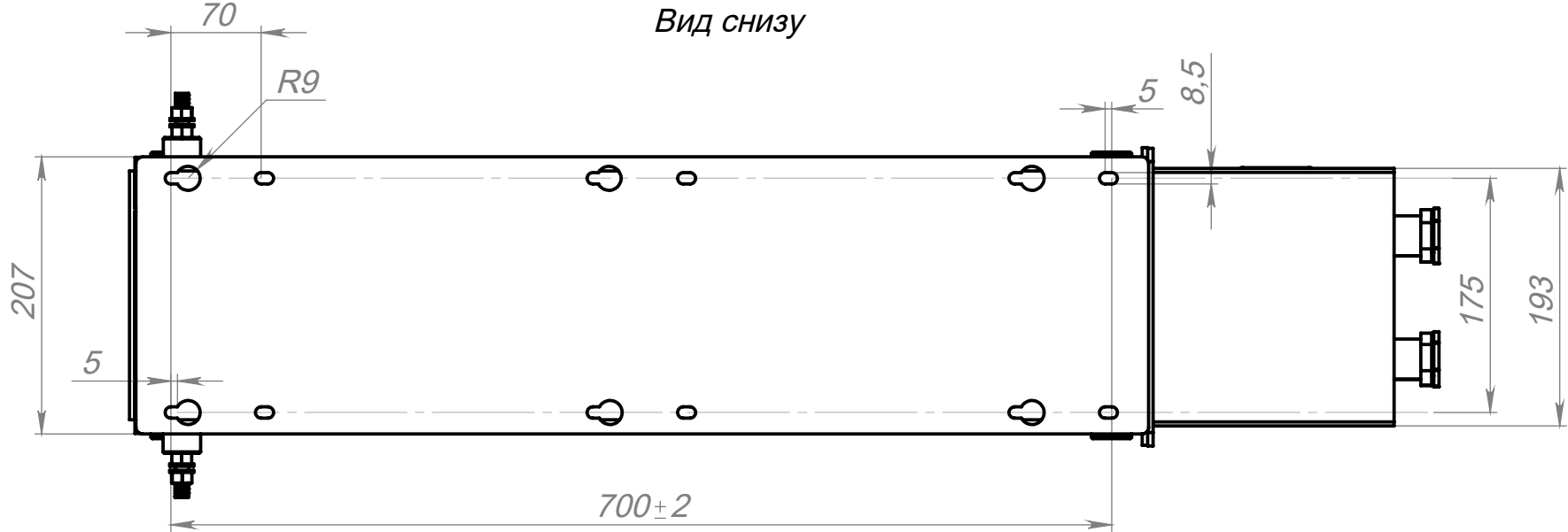
Вид снизу
