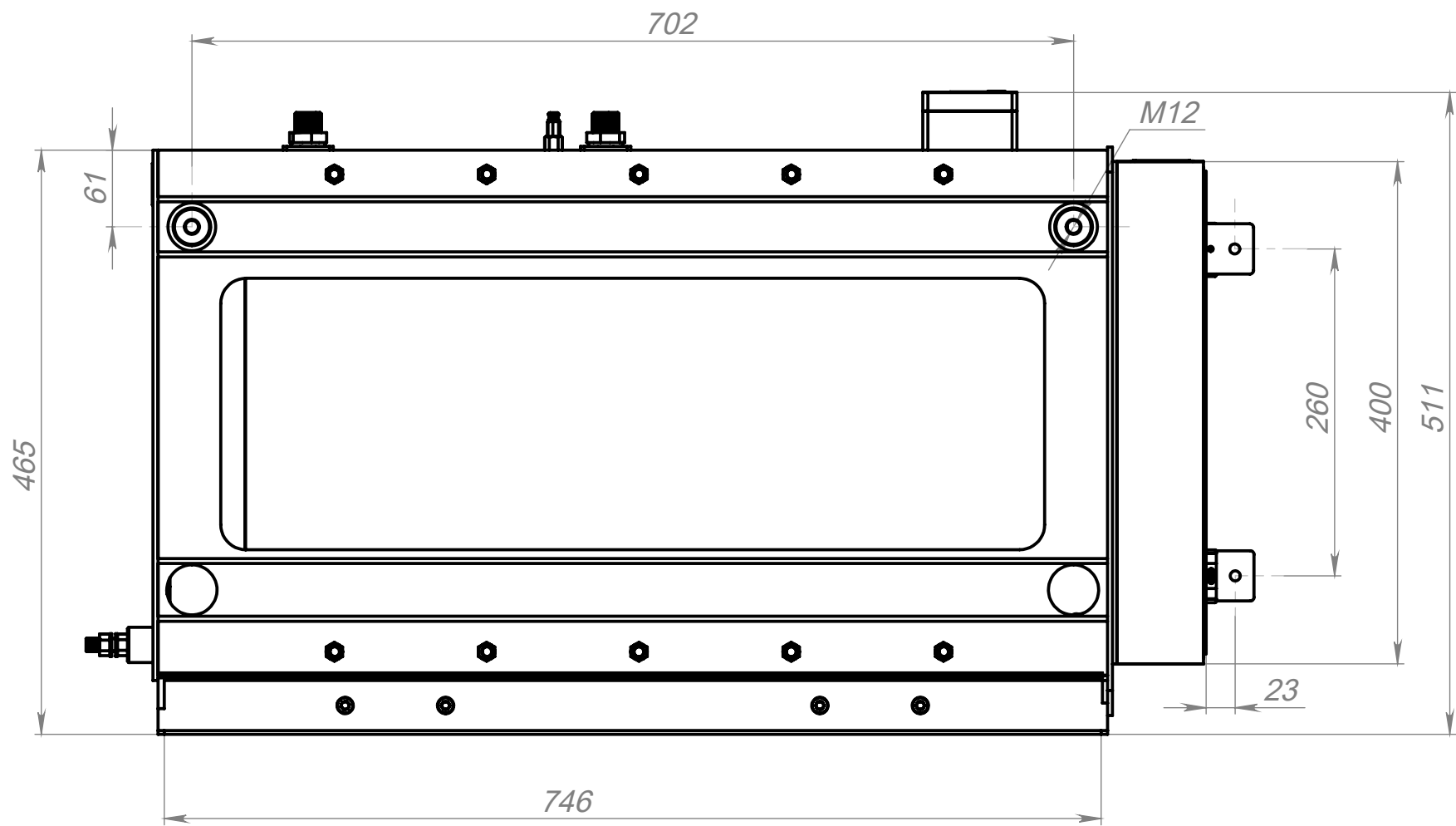
Вид спереди
