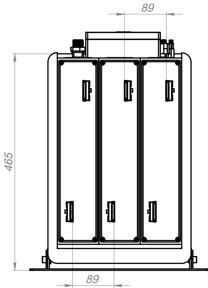
Вид справа
