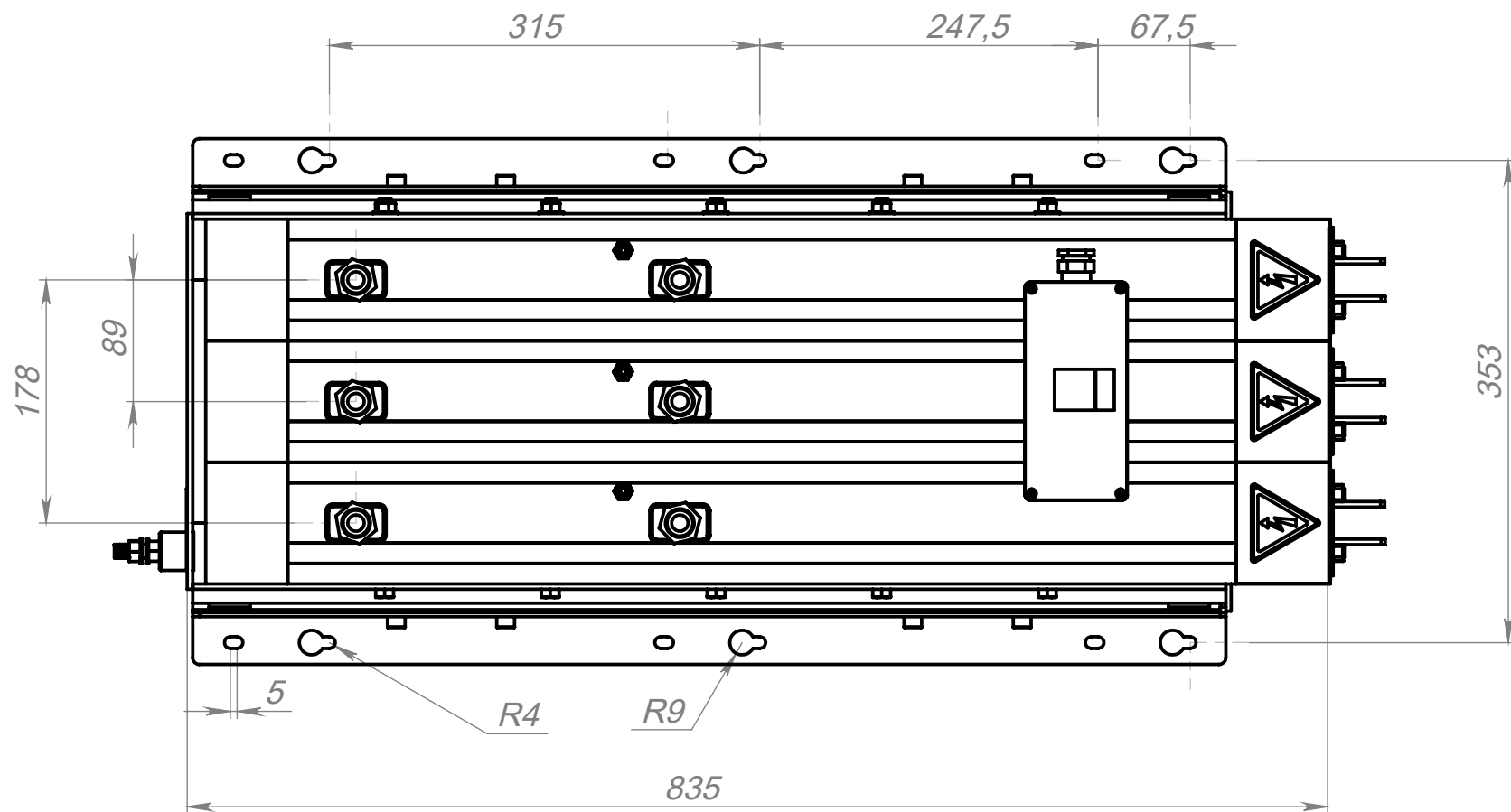
вид сверху
