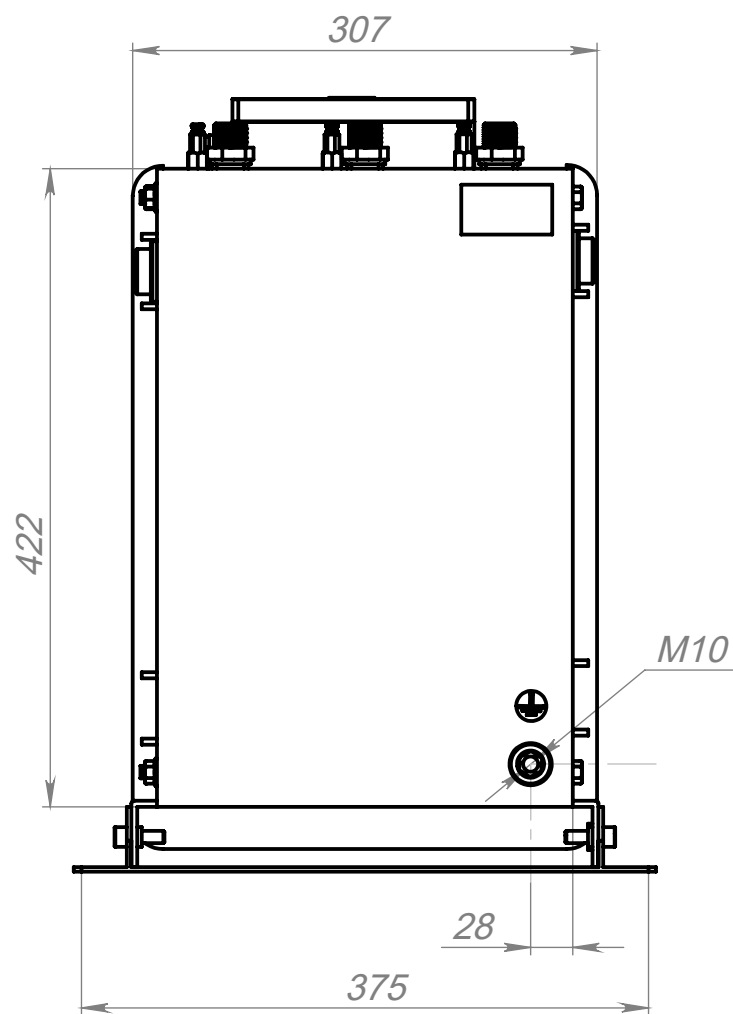
Вид слева
