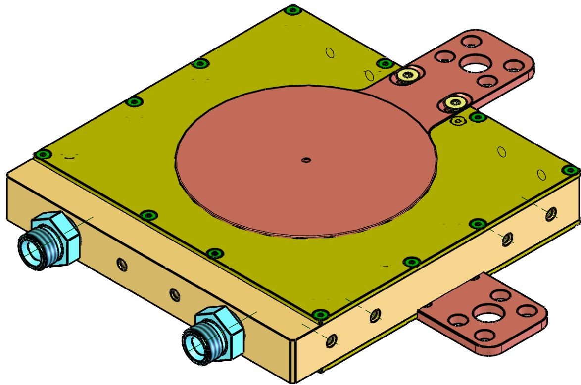
Вид К (1 : 2)
