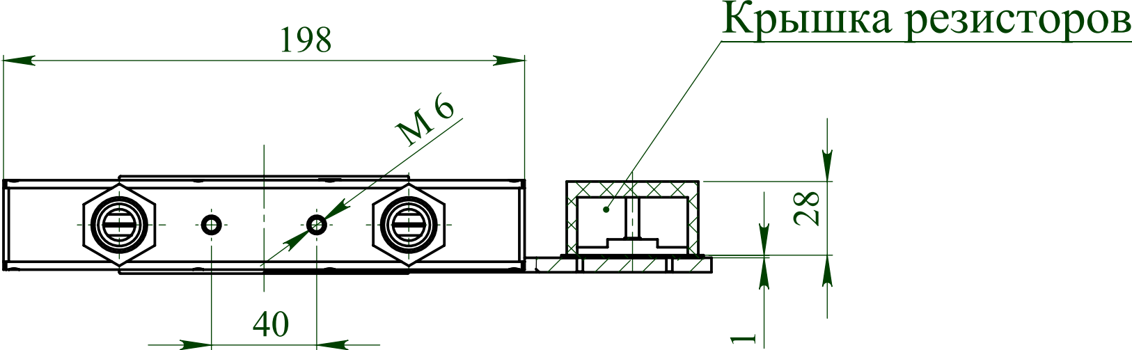
Вид К (1 : 2)
