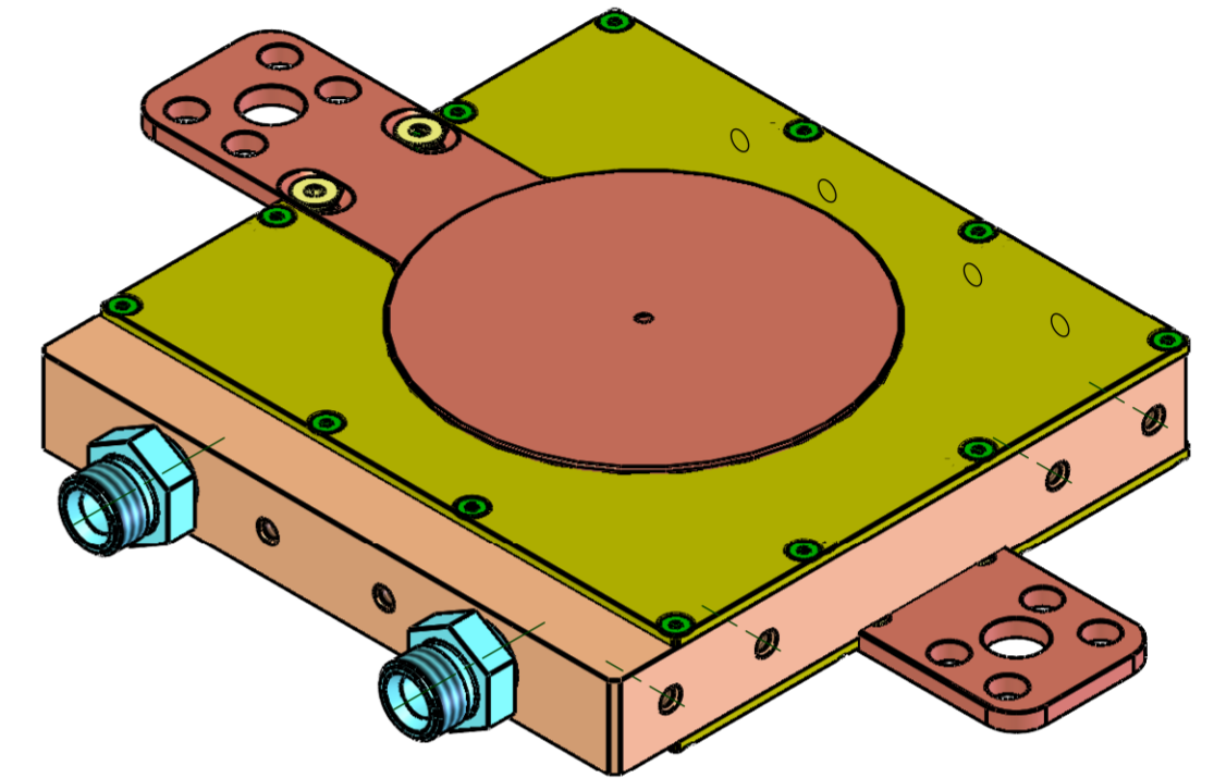
Вид К (1 : 2)
