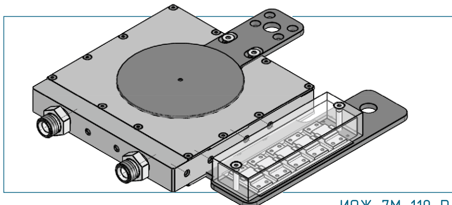
ИОЖ-7М-110-Р
